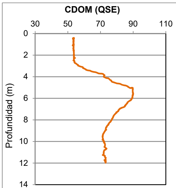
Figura 5. Perfil vertical de la conductividad y la materia orgánica cromofórica.
