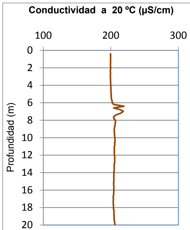
Figura 5. Perfil vertical de la conductividad.
