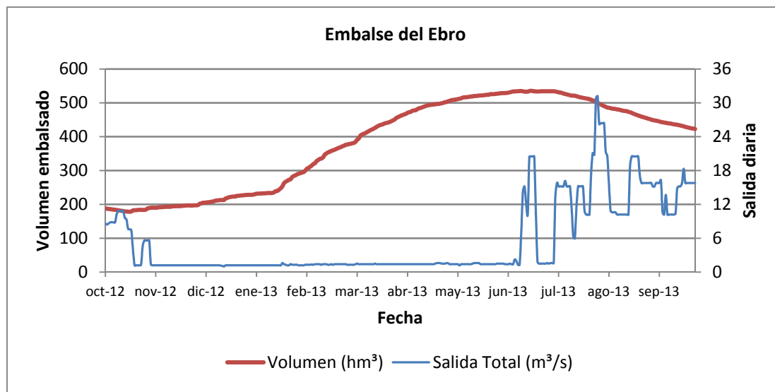
Figura 1. Volumen embalsado y salida durante el año hidrológico 2012-2013.
